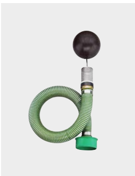
Retentionsdrossel mit Endkappe
